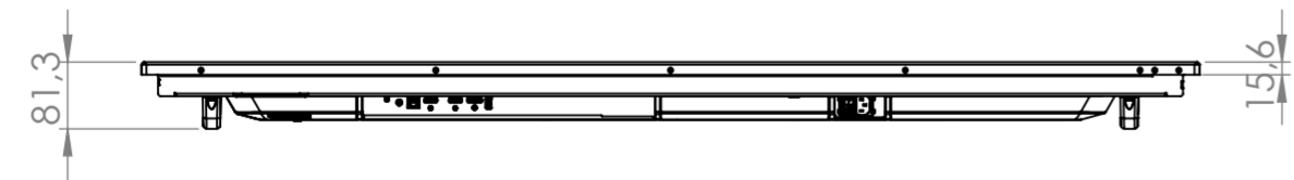
Bottom View Scale: 1:10
