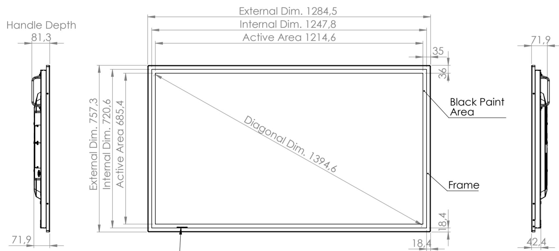
Front View Scale: 1:10
