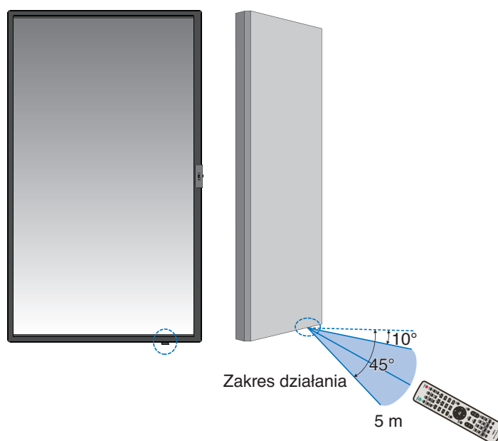
Zakres działania w orientacji pionowej
