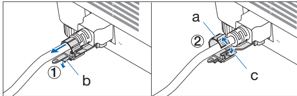
a: Klemme/b: Knopf (Netzkabelsicherung)/c: Knopf (Klemme)
