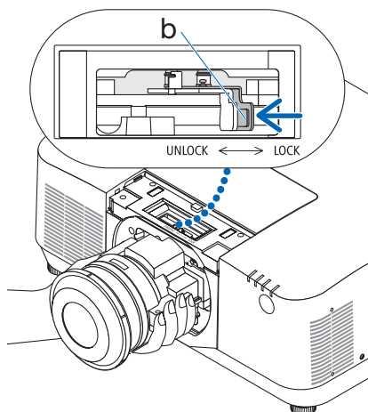
b: Objektivsperrhebel
