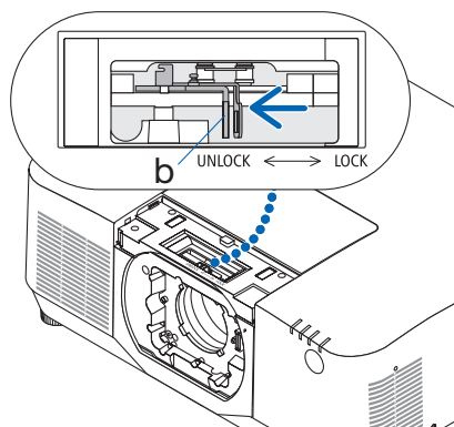
b: Objektivsperrhebel
