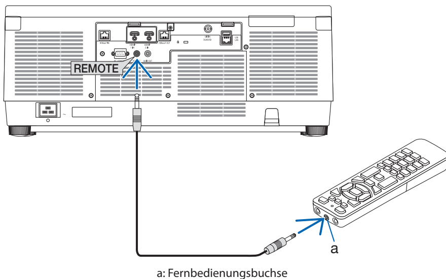
a: Fernbedienungsbuchse
